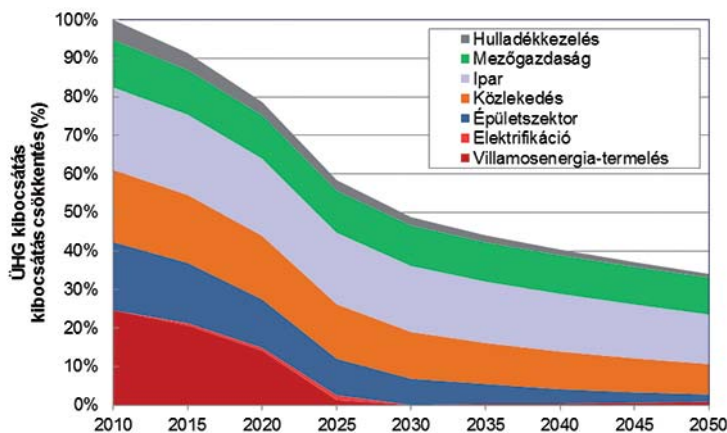
8. ábra. A szektorális minimum ÜHG-kibocsátási pályák nemzetgazdasági összesítése Forrás: NÉS-2b, 186.
