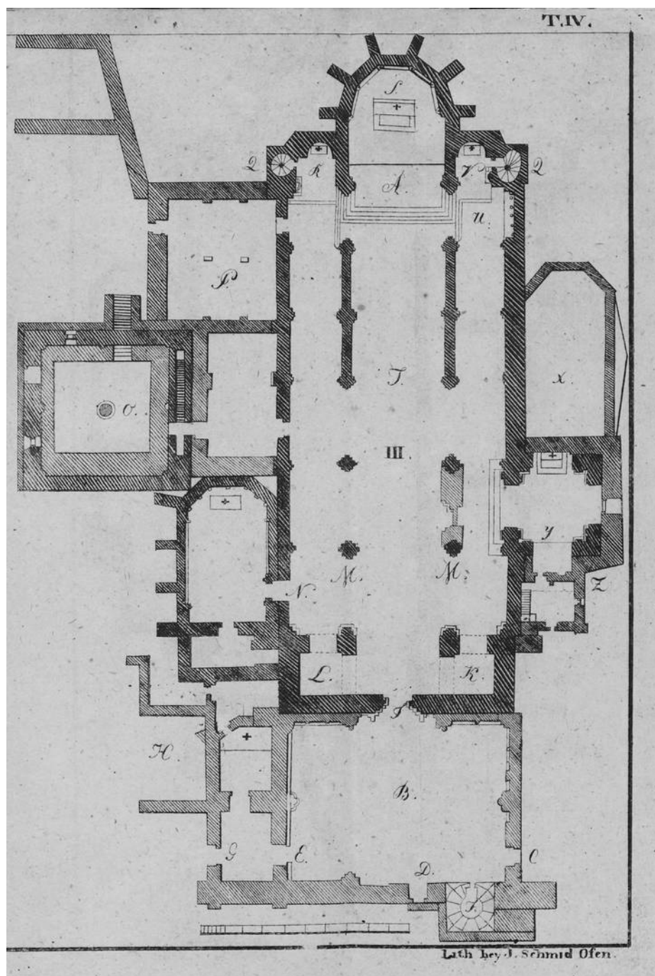
Máthes János 1827-ben közölt litografált székesegyház alaprajza (MÁTHES: 1827, Tab. IV.).
